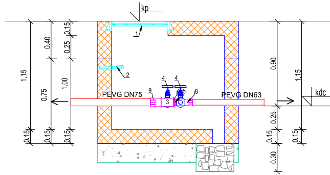
PRESJEK 1-1
