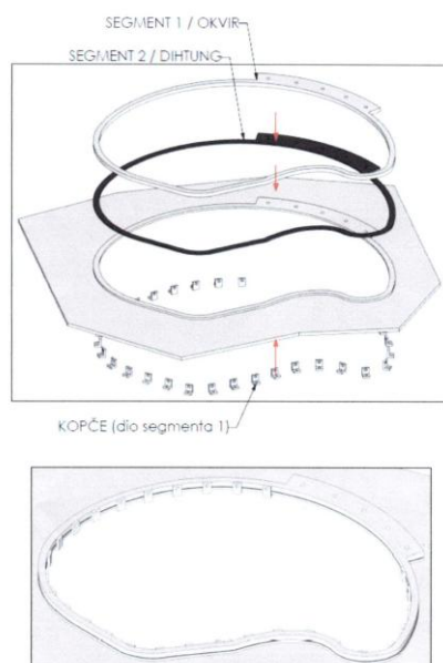
5 - Sklopni crtež
