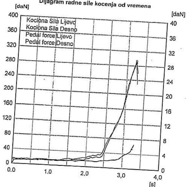
Dijagram radne sile kocenja od vremena
