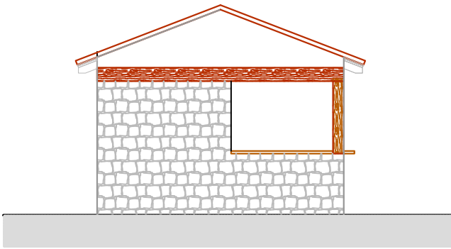
ZAPADNA FASADA
