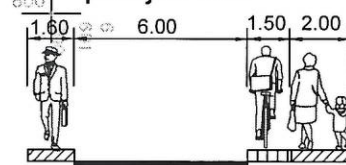
presjek 4-4
