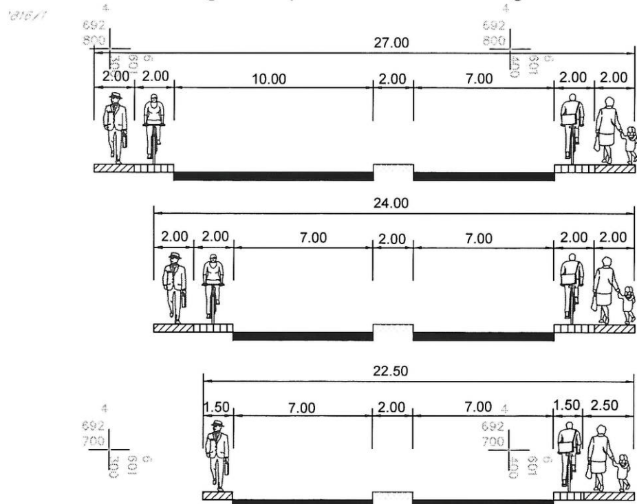
presjek 1-1
