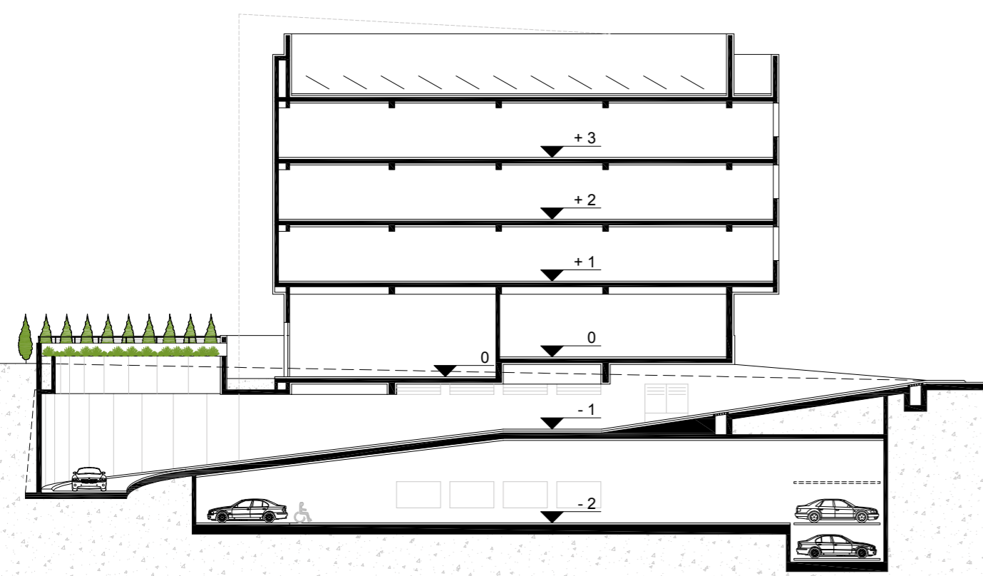
PRESJEK KROZ RAMPU
