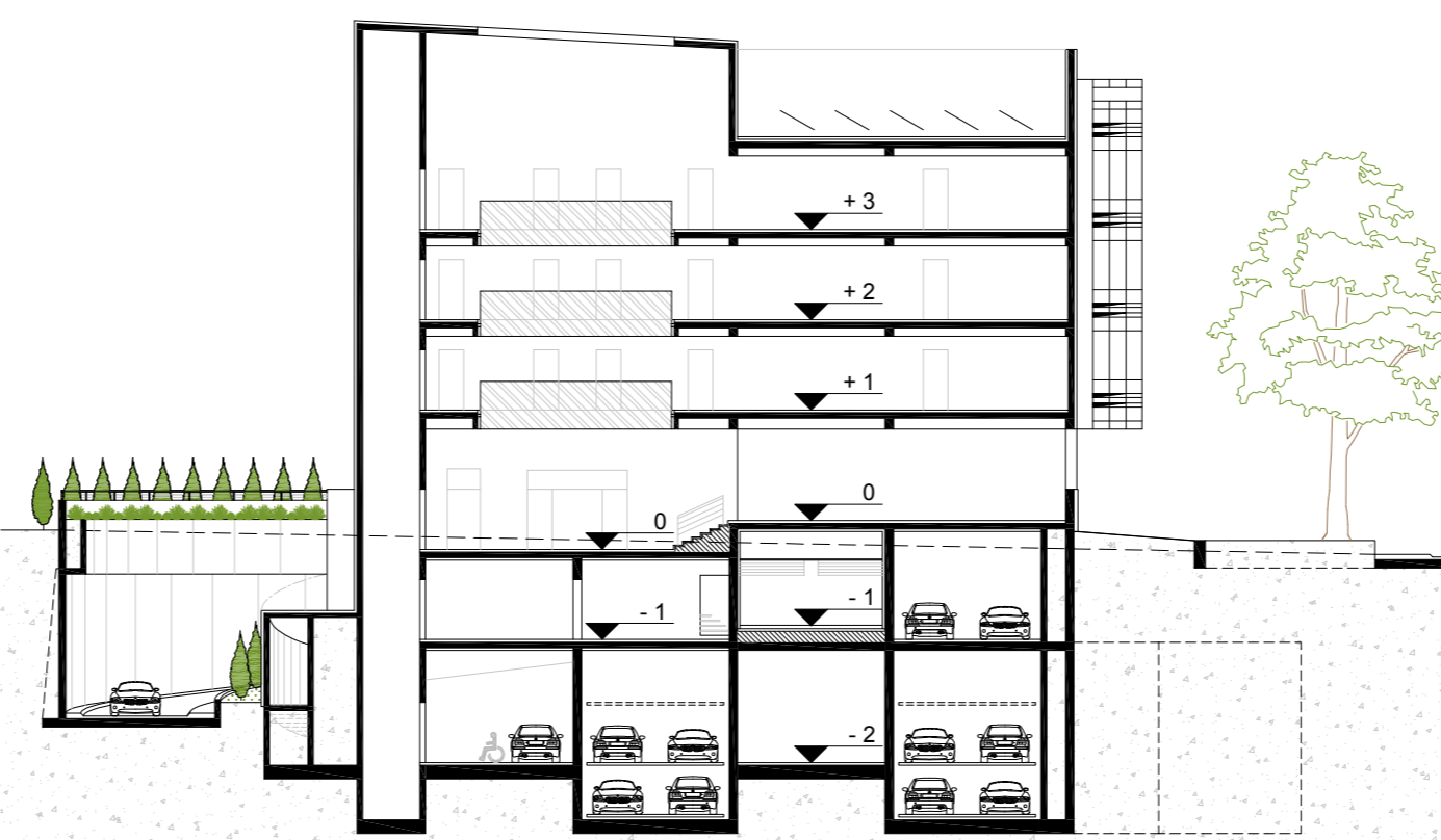
PRESJEK KROZ ATRIJUM
