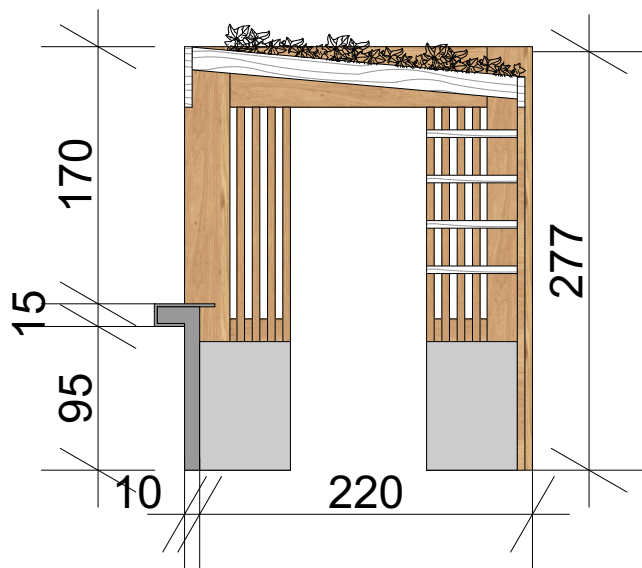
presjek 1-1
