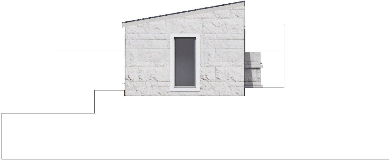
BOČNI IZGLED
