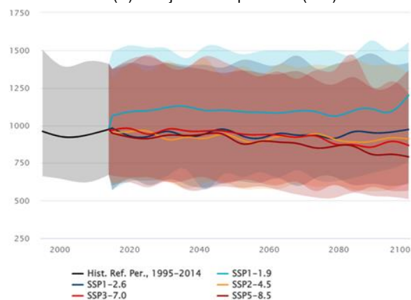
Slika 4.4 (A-D) Uticaj klimatskih promjena na padavine u Crnoj Gori
