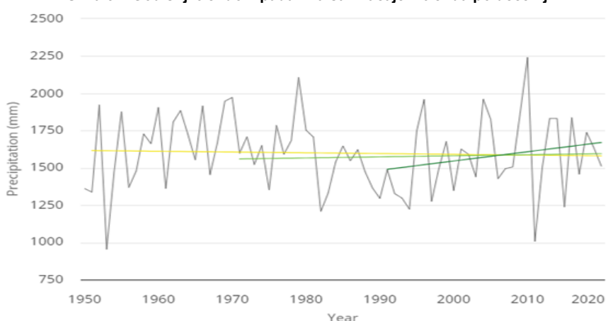
Slika 3.2 Godišnji trendovi padavina sa značajem trenda po deceniji
