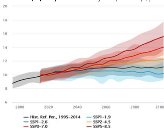
Slika 3.3 (A-D) Uticaj klimatskih promjena na temperature u Crnoj Gori
