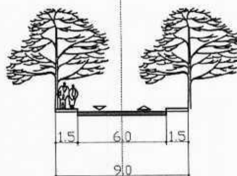
presjek 4-4
