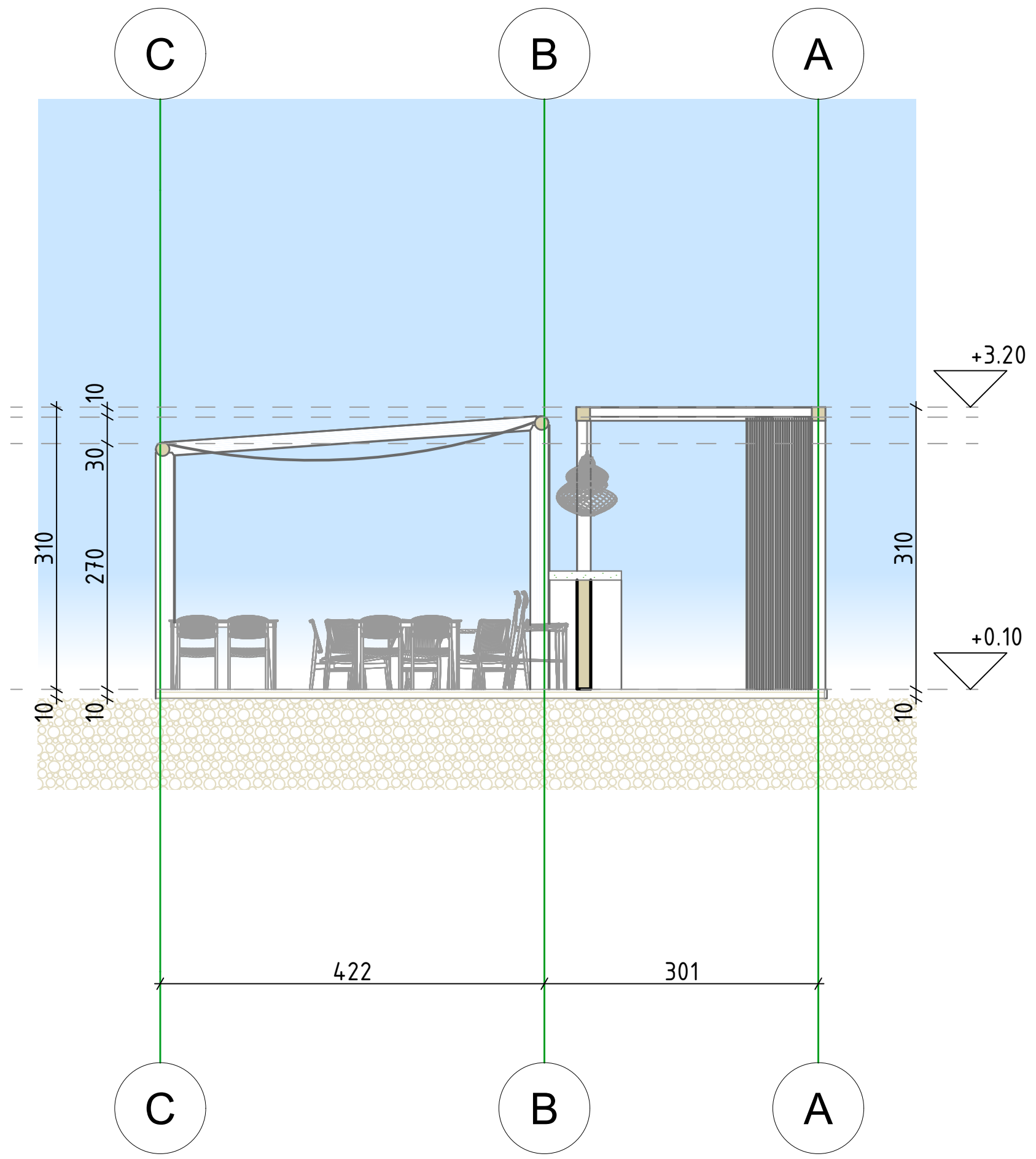
PRESJEK B-B
