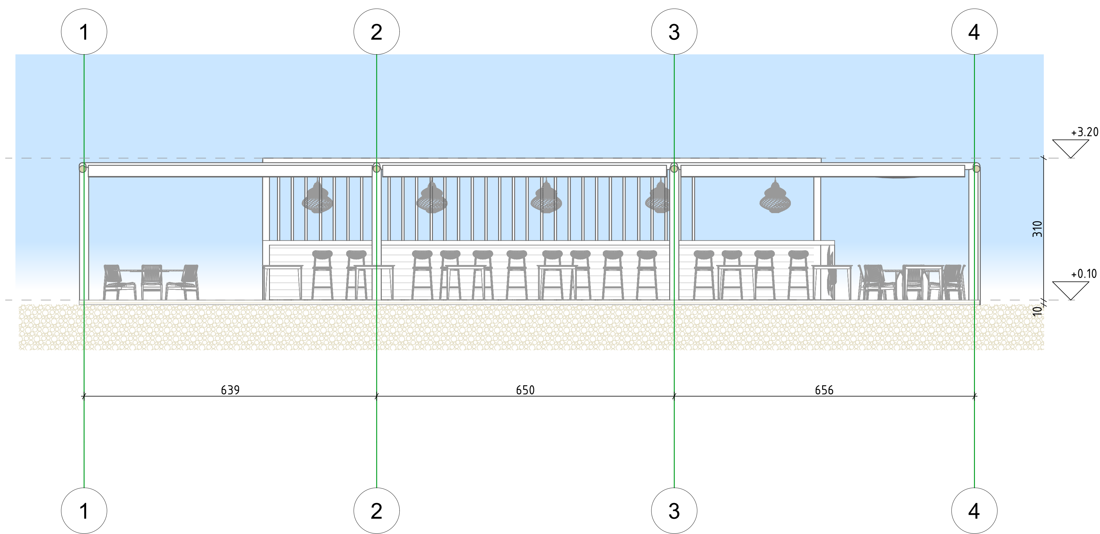
PRESJEK B-B
