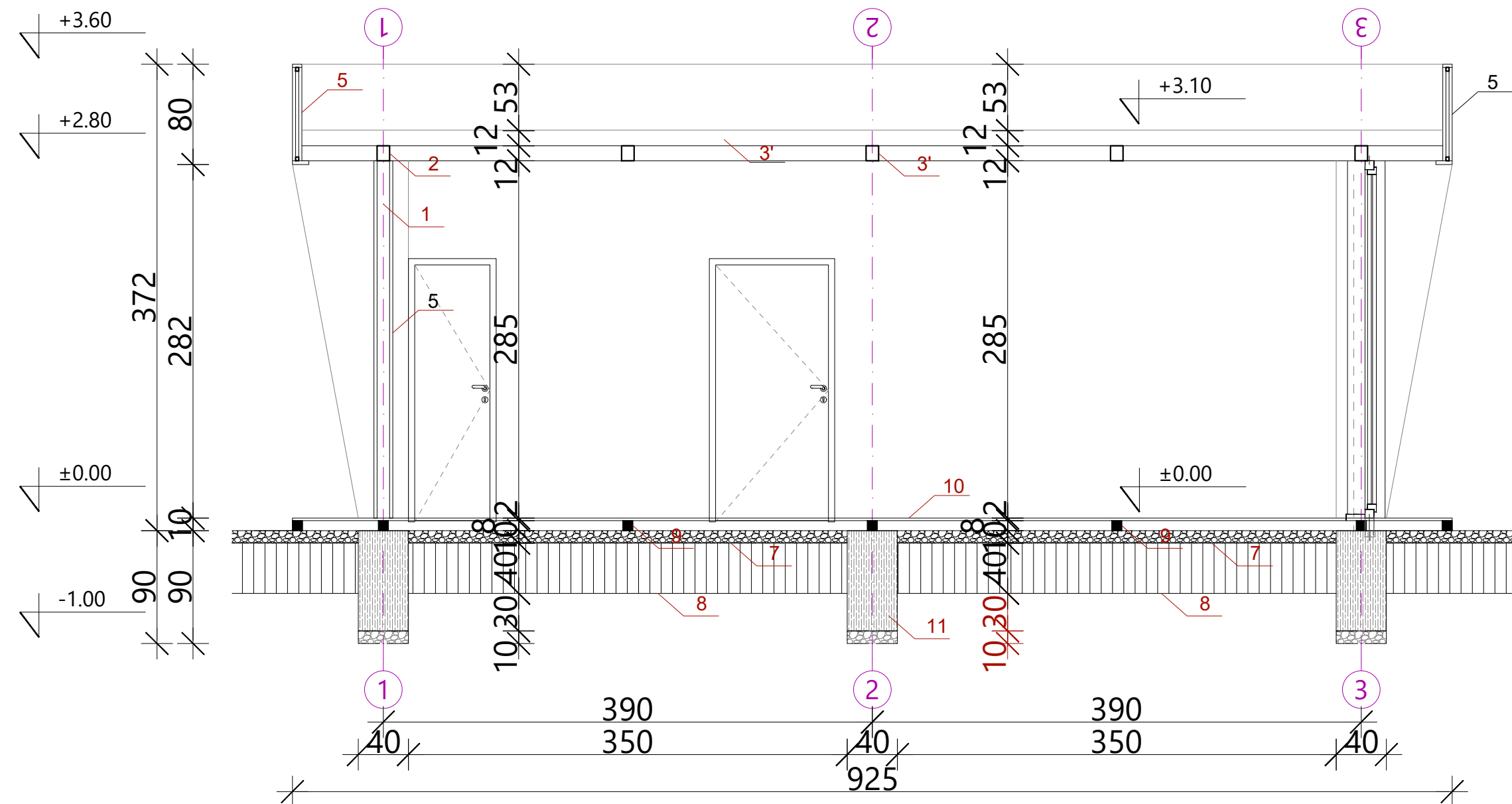
PRESJEK 2-2
