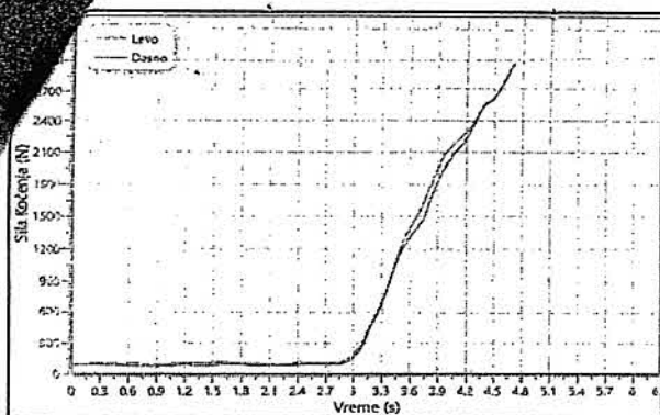
Parkirna kočnica
