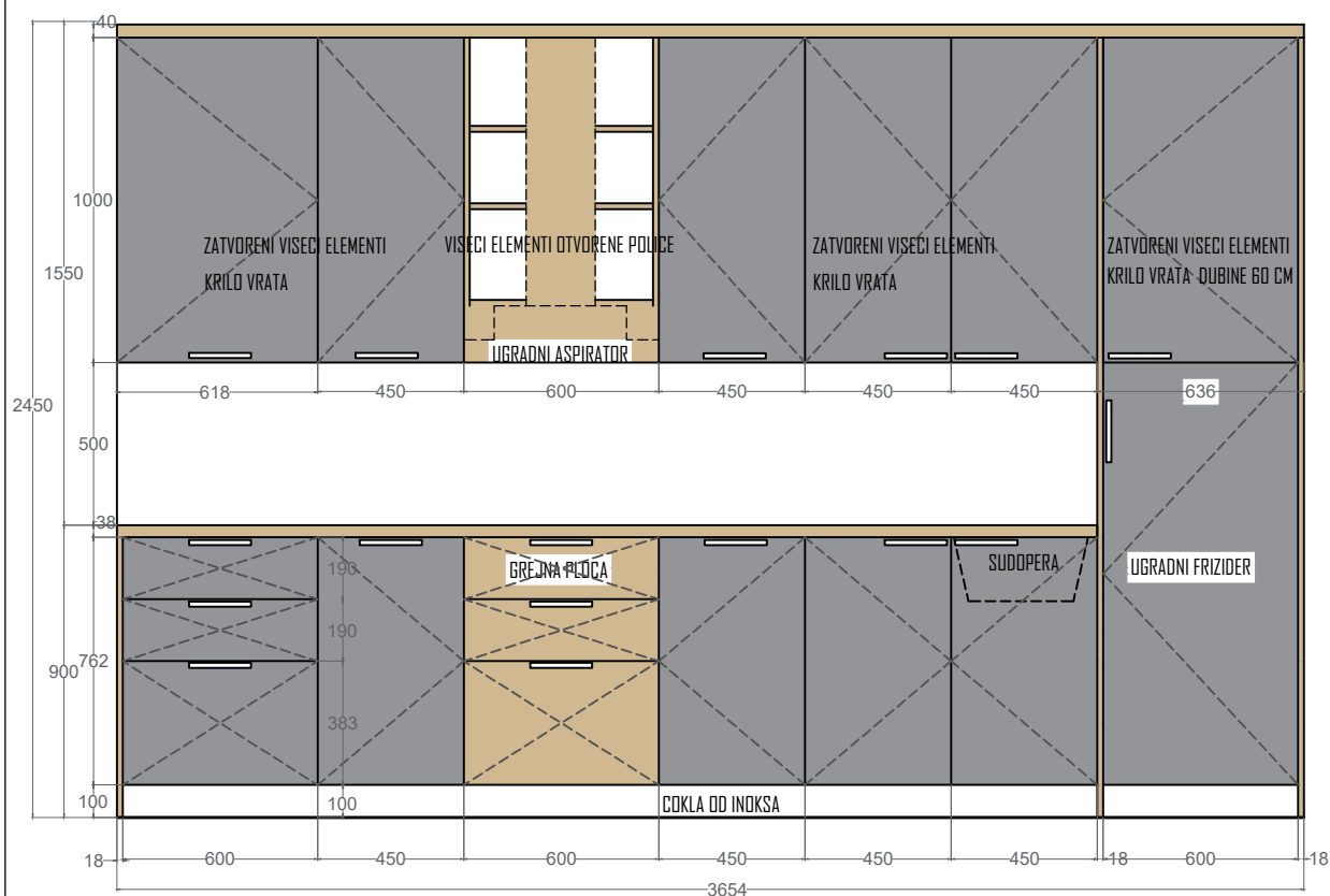
POGLED I-I
