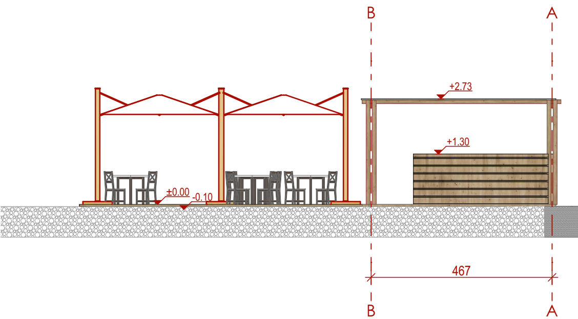
B Elevation 1:100
