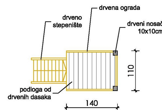
OSNOVA
