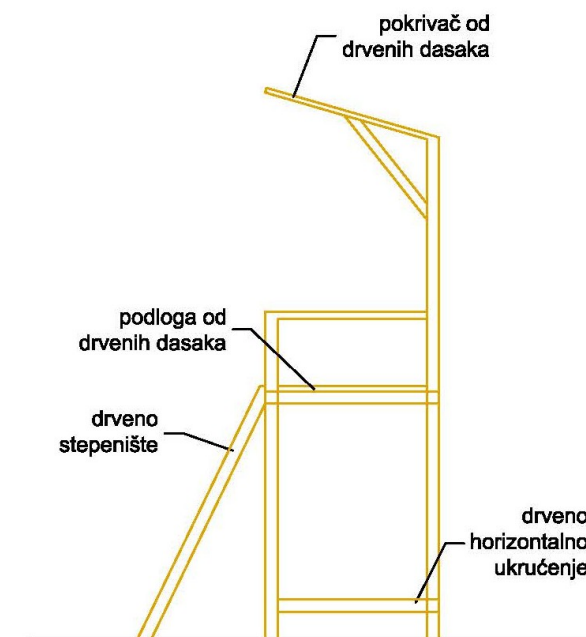
IZGLED A
