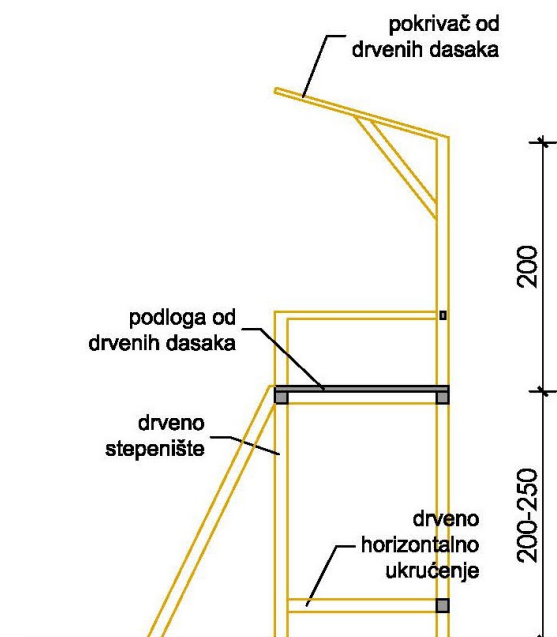
PRESJEK
