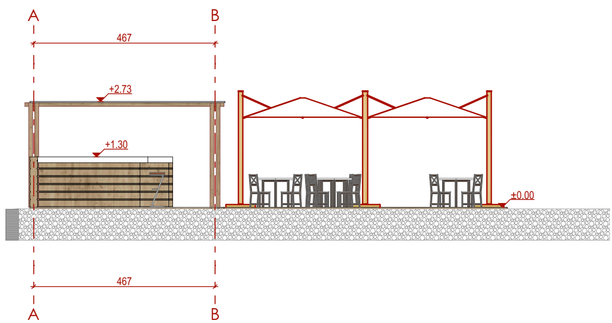
C Elevation 1:100
