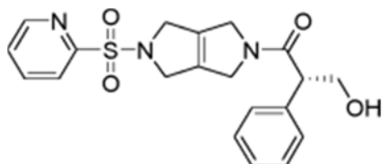
(2S)-3-hidroksi-2-fenil-1-[5-(piridin-2-sulfonyl)-1H,2H,3H,4H,5H,6H-piolo[3,4-c]pirol-2-il]propan-1-on
