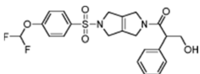
1-(5-((4-(difluorometoksi)fenil)sulfonyl)-3,4,5,6-tetrahidropiolo[3,4-c]pirol-2(1H)-il)-3-hidroksi-2-fenilpropan-1-on
