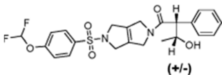
(2R,3R i 2S,3S)-1-(5-((4-(difluorometoksi)fenil)sulfonil)-3,4,5,6-tetrahidropirol[3,4-c]pirol-2(1H)-il)-3-hidroksi-2-fenilbutan-1-on
