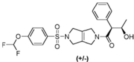
(2S,3R i 2R,3S)-1-(5-((4-(difluorometoksi)fenil)sulfonil)-3,4,5,6-tetrahidropirol[3,4-c]pirol-2(1H)-il)-3-hidroksi-2-fenilbutan-1-on
