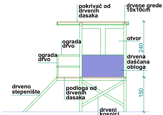
PRESJEK 1-1
